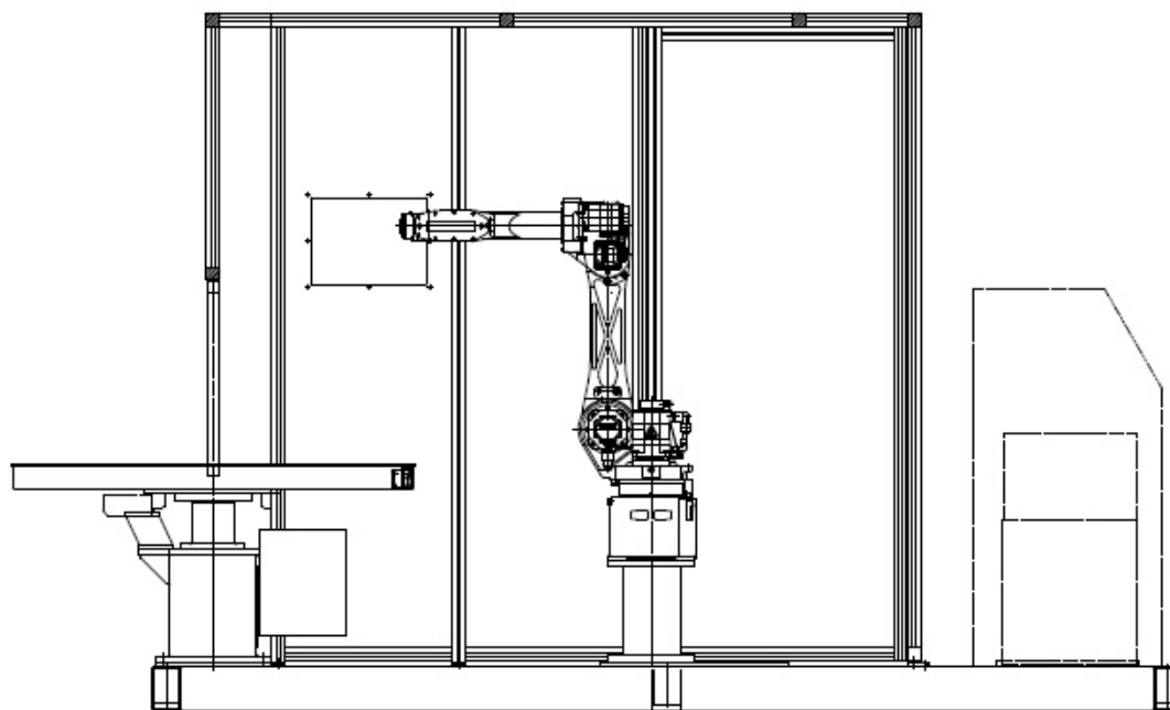
Figura 1- Sistemas Weldpro
